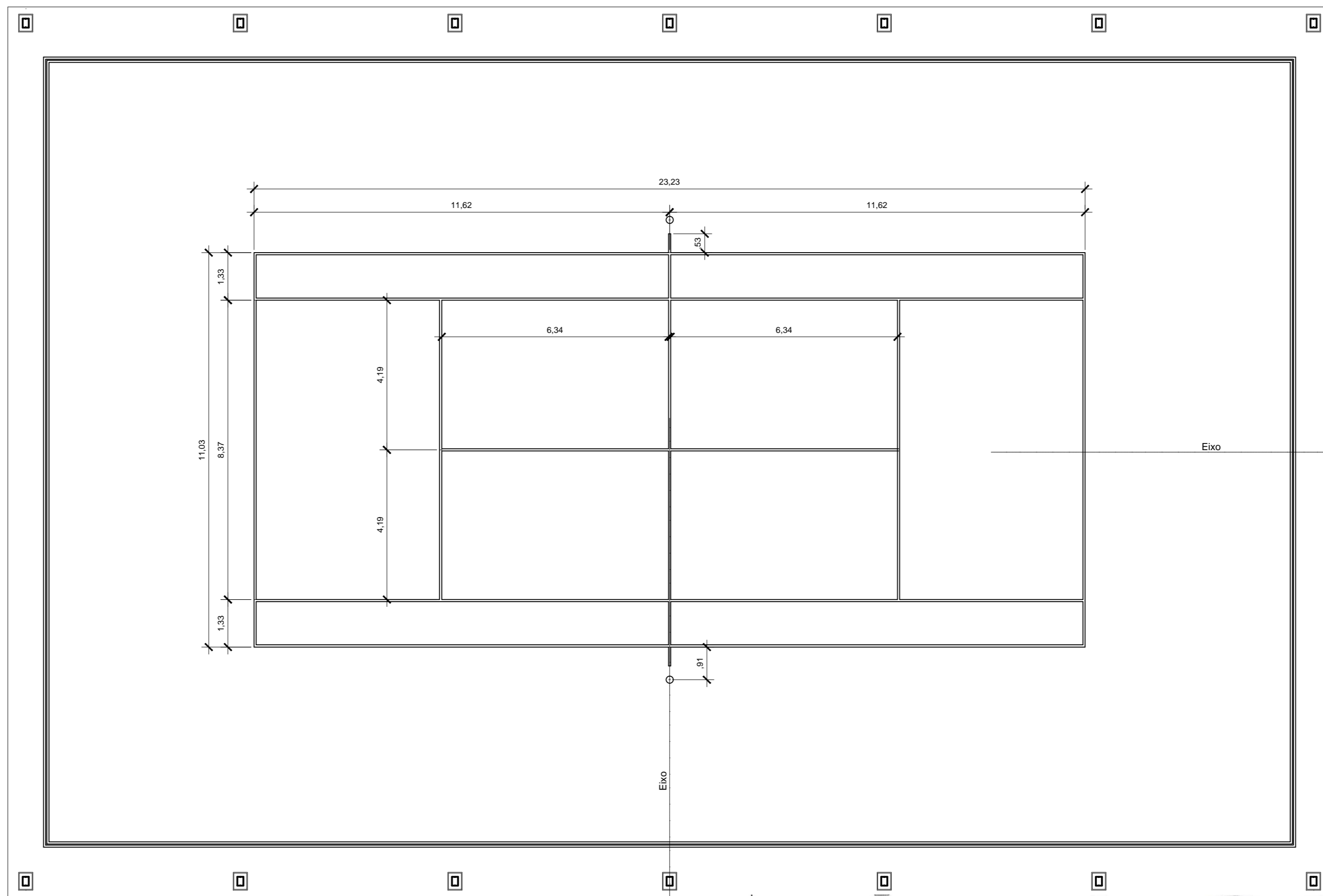
DEMARCAÇÃO TÊNIS 156,49 m - Branco 1:100
